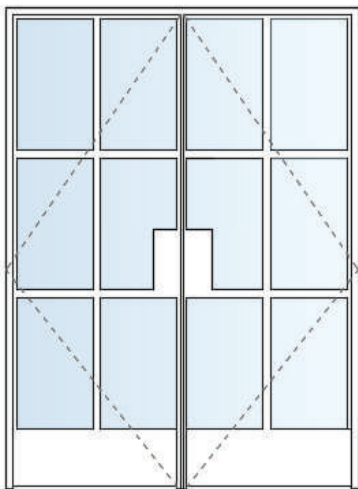
9 6080 Double Door Custom 2x3 Light
